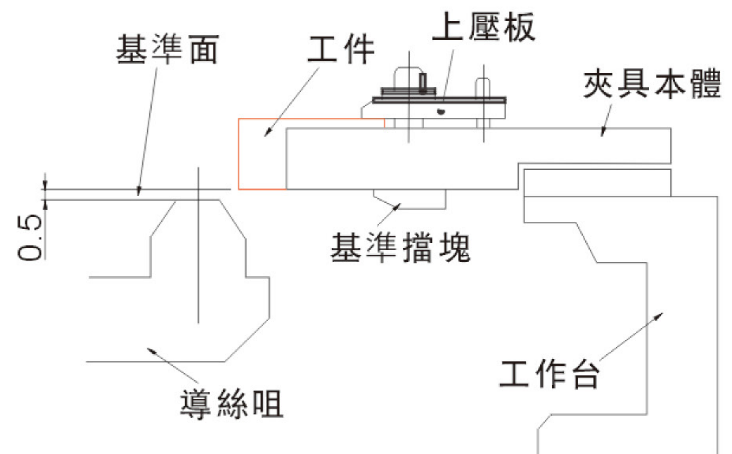
裝夾位置關係圖 夾具與導絲嘴的位置關係
